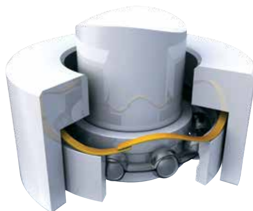
G. Roulements précontraints
