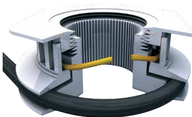
B. Joint d'étanchéité mécanique
