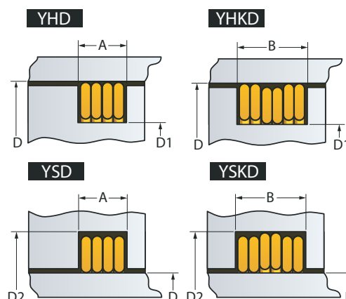
Dimensions des produits Toutes les dimensions sont exprimées en pouces sauf spécification contraire.
